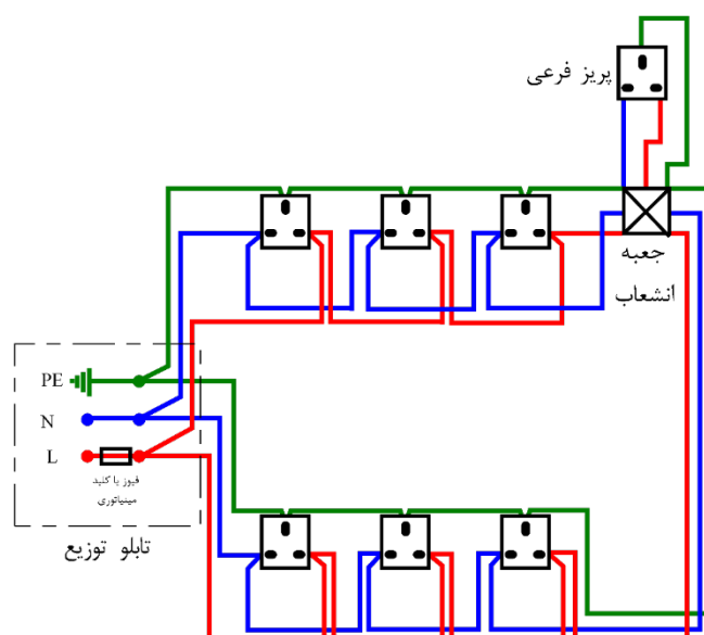
شکل ۴-۴- سیستم سیم‌کشی حلقوی مدار پریشها
