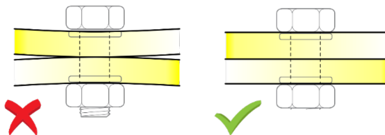
شکل ۶-۲۴- فشار سطح تماس شیشه‌ها
