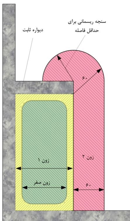
شکل ۴-۸- ابعاد زون‌ها: دید از بالای وان حمام با دیواره ثابت
